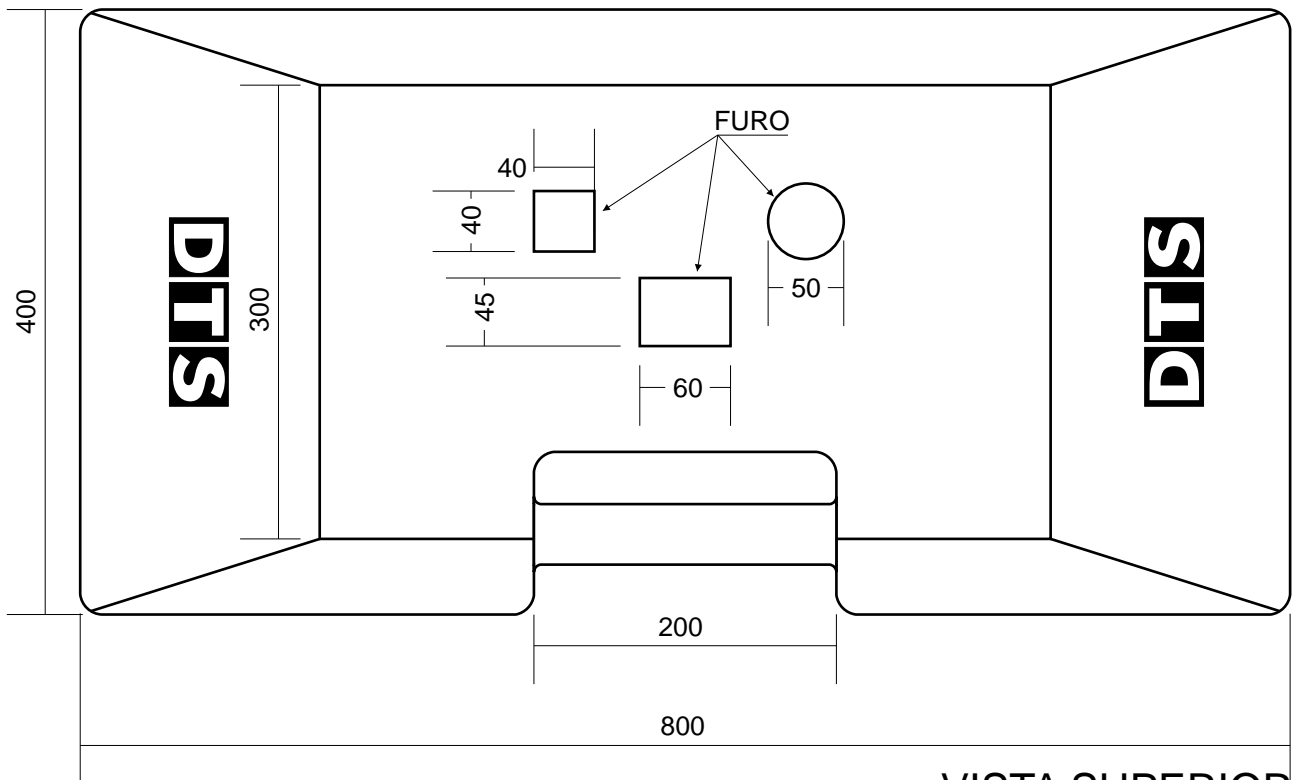
VISTA SUPERIOR
