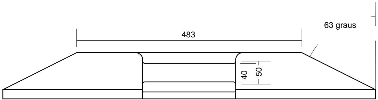
VISTA LATERAL
